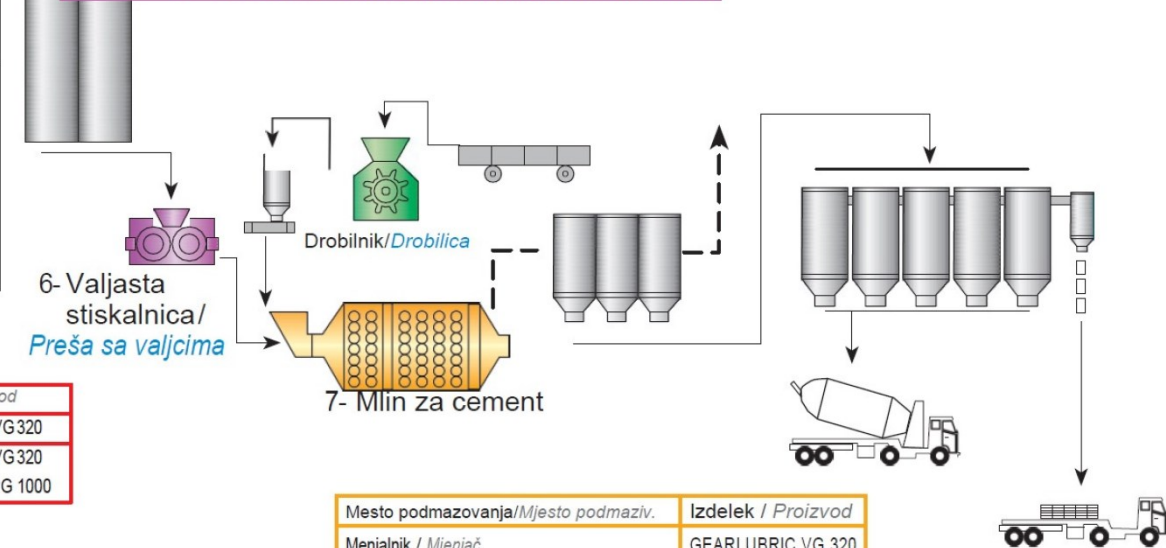
6- VALJASTA STISKALNICA/PREŠA SA VALJCIMA
